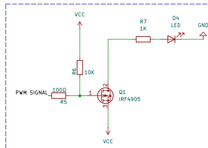
P Type - MOSFET Switchig
