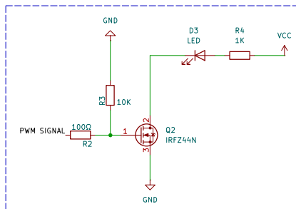
N Type - MOSFET Switchig
